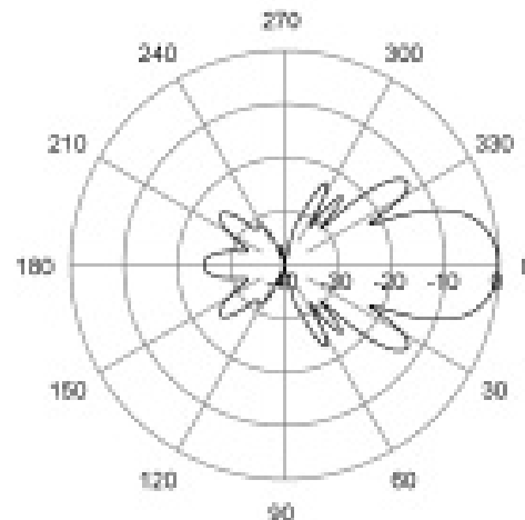
E-Plane | 455 MHz
