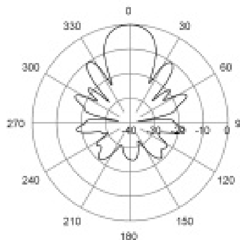
H-Plane | 455 MHz
