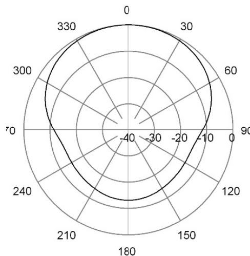
H-Plane | 73 MHz
