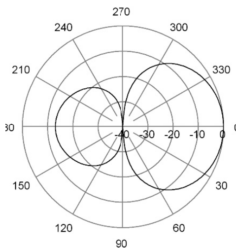
E-Plane | 78 MHz
