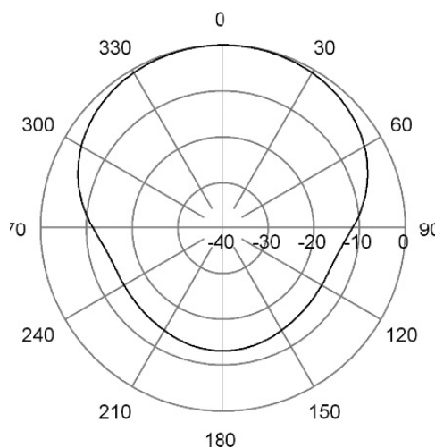
H-Plane | 78 MHz
