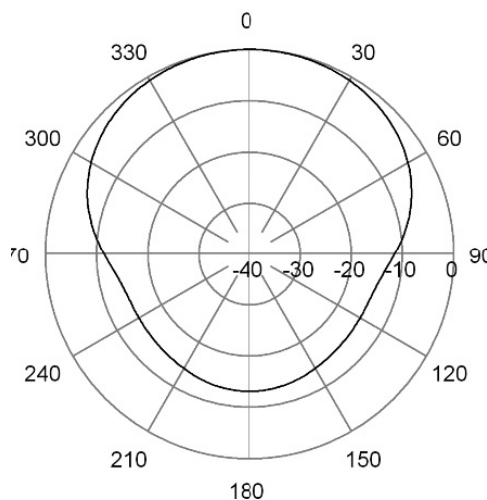
H-Plane | 102 MHz
