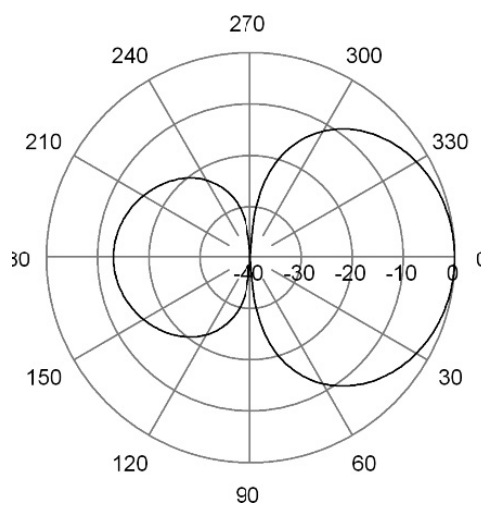
E-Plane | 120 MHz
