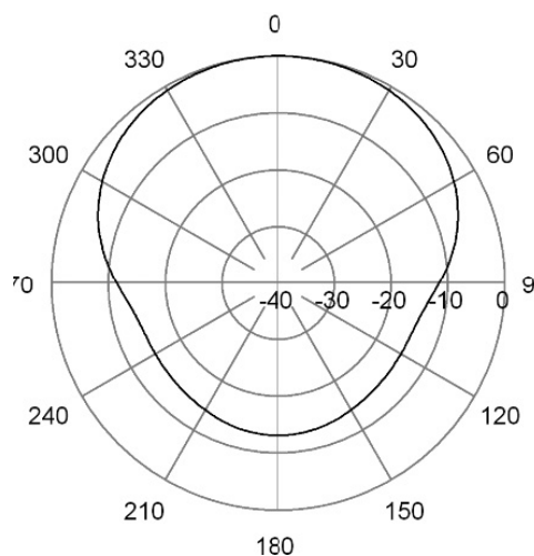
H-Plane | 120 MHz
