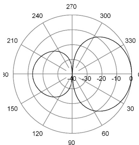
E-Plane | 185 MHz
