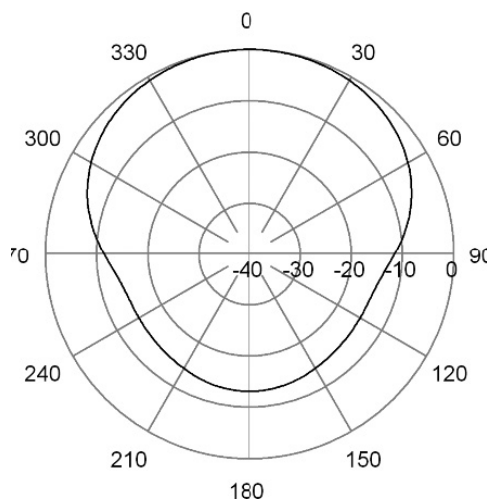
H-Plane | 185 MHz
