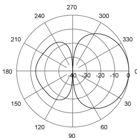
E-Plane | 153 MHz
