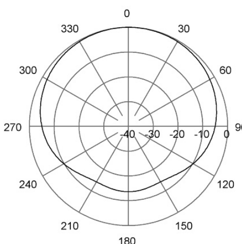
H-Plane | 153 MHz
