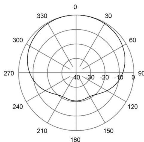
H-Plane | 152 MHz
