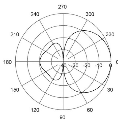
E-Plane | 152 MHz
