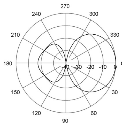
E-Plane | 160 MHz
