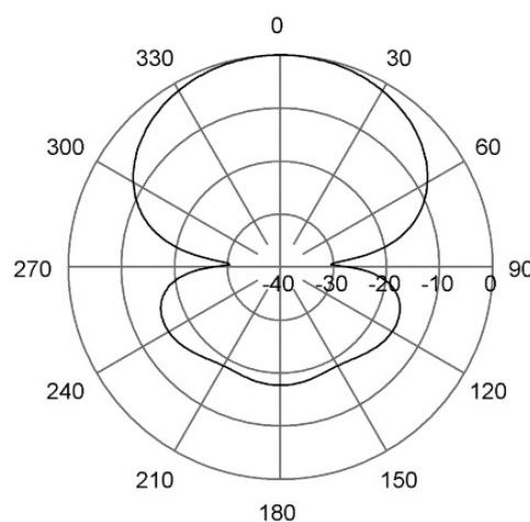
H-Plane | 160 MHz
