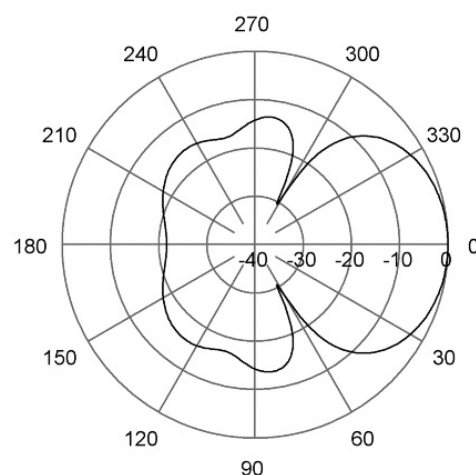
H-Plane | 390 MHz
