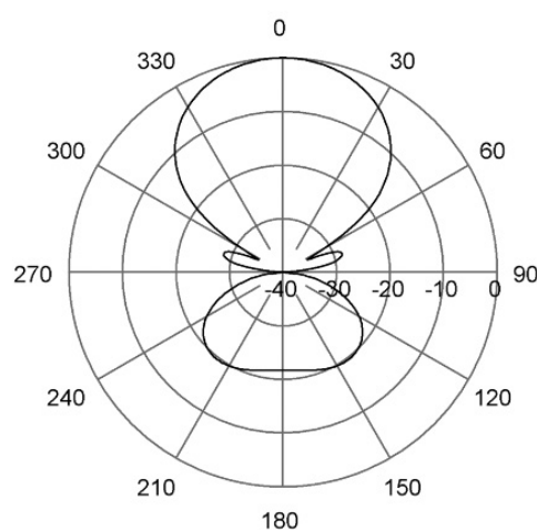
E-Plane | 390 MHz
