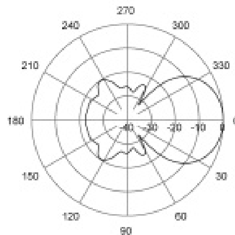
E-Plane | 436 MHz
