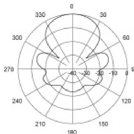
H-Plane | 436 MHz
