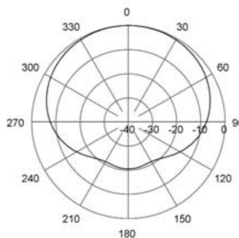
H-Plane | 144 MHz
