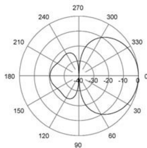
E-Plane | 160 MHz
