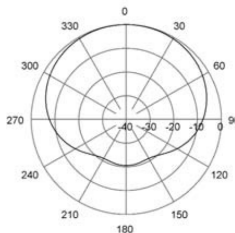
H-Plane | 160 MHz
