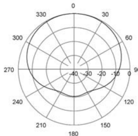
H-Plane | 210 MHz
