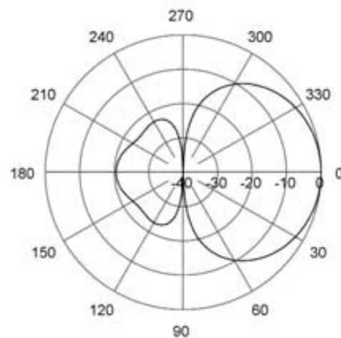
E-Plane | 210 MHz
