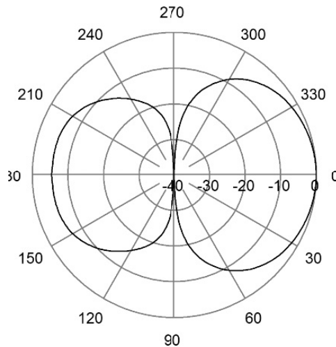
E-Plane | 56 MHz
