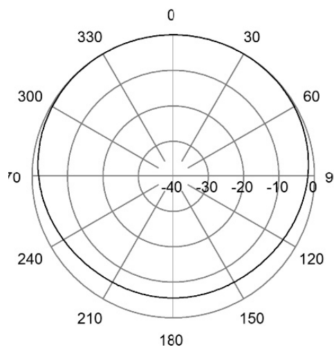
H-Plane | 85 MHz
