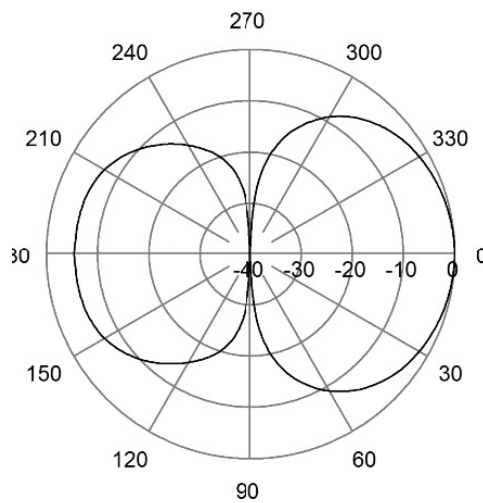
E-Plane | 85 MHz
