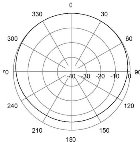
H-Plane | 148 MHz
