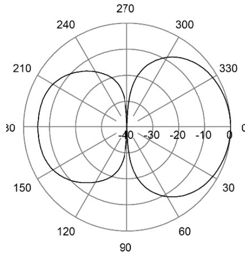
E-Plane | 148 MHz
