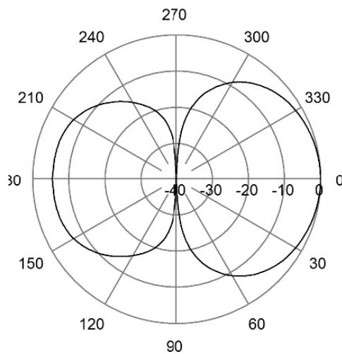
E-Plane | 355 MHz
