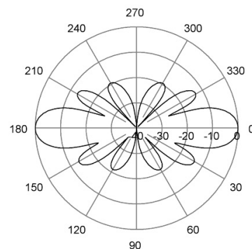
E-Plane | 148 MHz
