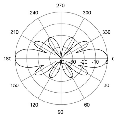
E-Plane | 159 MHz
