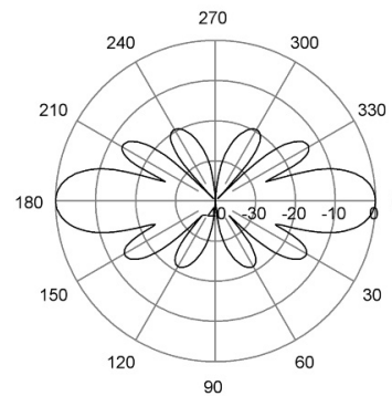
E-Plane | 173 MHz
