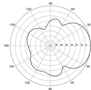
H-Plane | 405 MHz
