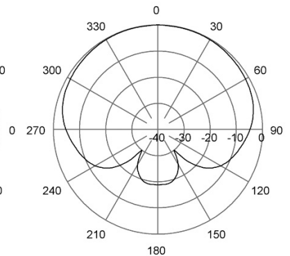
H-Plane | 182 MHz
