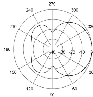
E-Plane | 182 MHz
