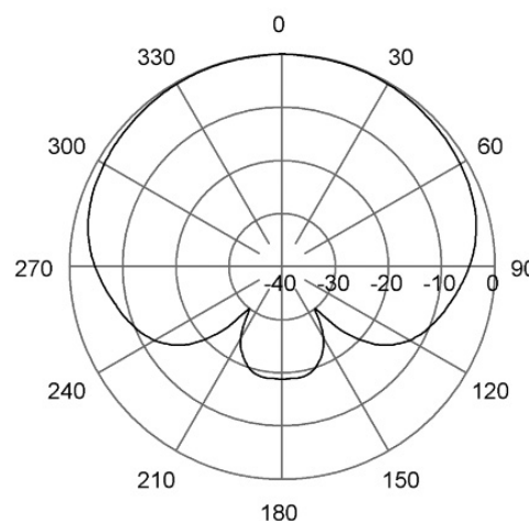
H-Plane | 460 MHz
