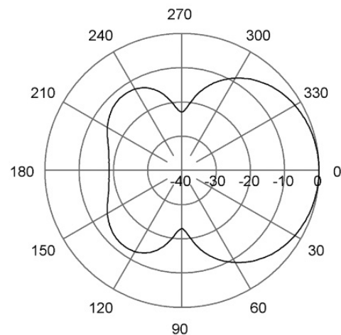
E-Plane | 460 MHz
