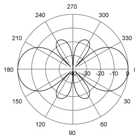
E-Plane | 150 MHz
