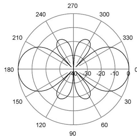
E-Plane | 184 MHz
