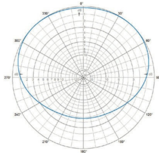
H-Plane | 127 MHz
