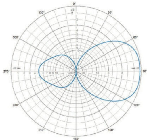
E-Plane | 127 MHz
